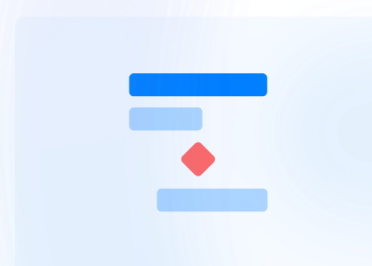
甘特图
