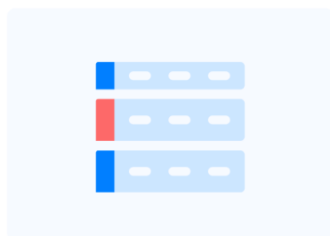
软件架构图
