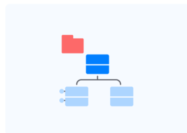
UML图
