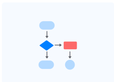
基本流程图
